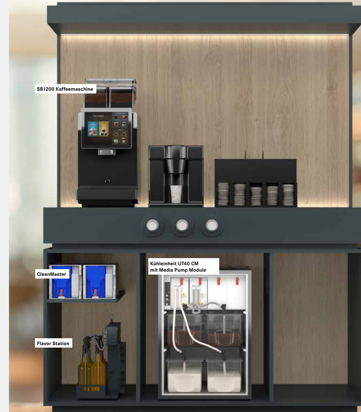
Möbiliar nicht Teil der Specialty Beverage Station von Franke - muss vom Kunden bereitgestellt werden.
